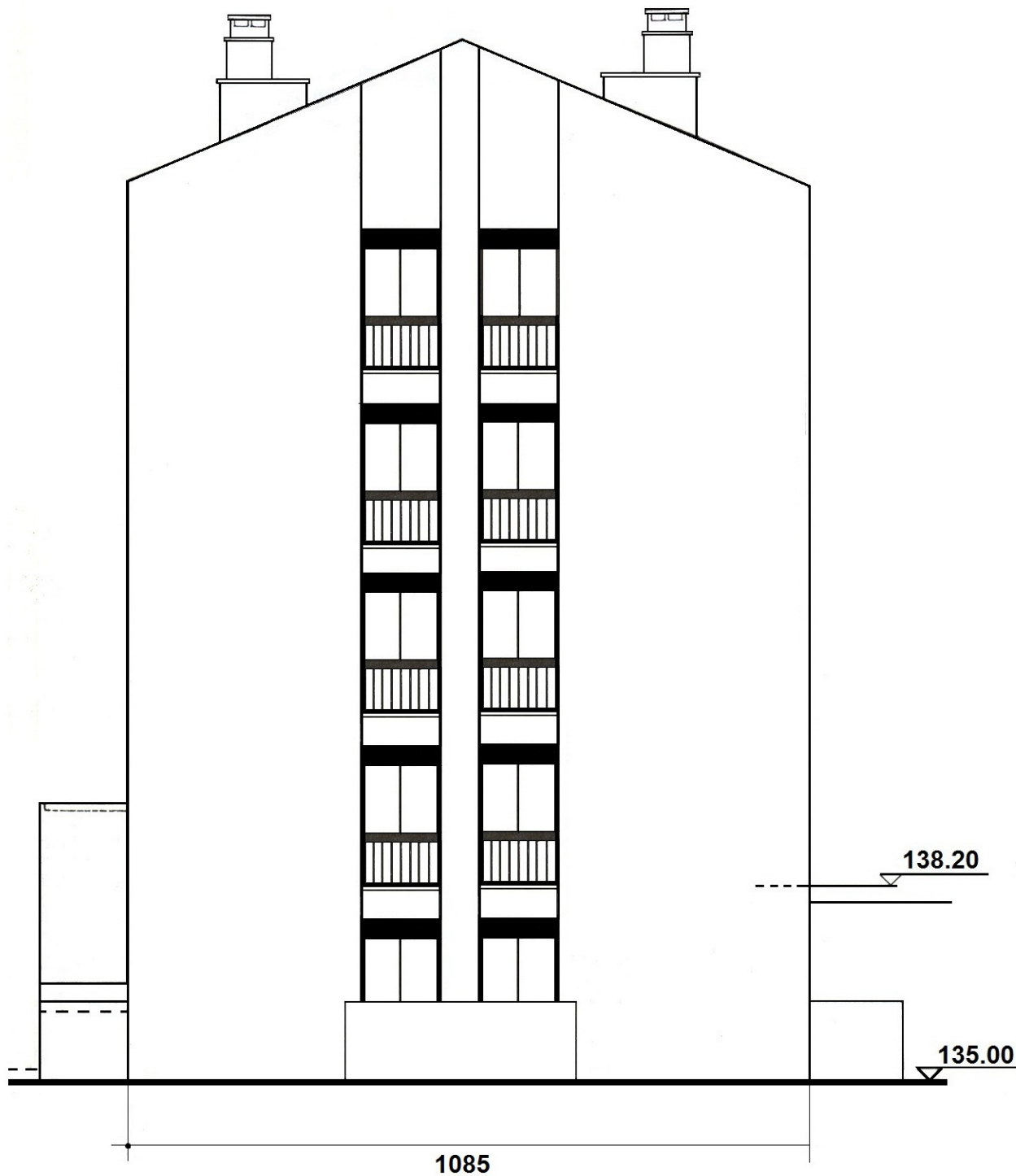
Alçado Sul do N° 1 da Praceta José Duro Massamá
